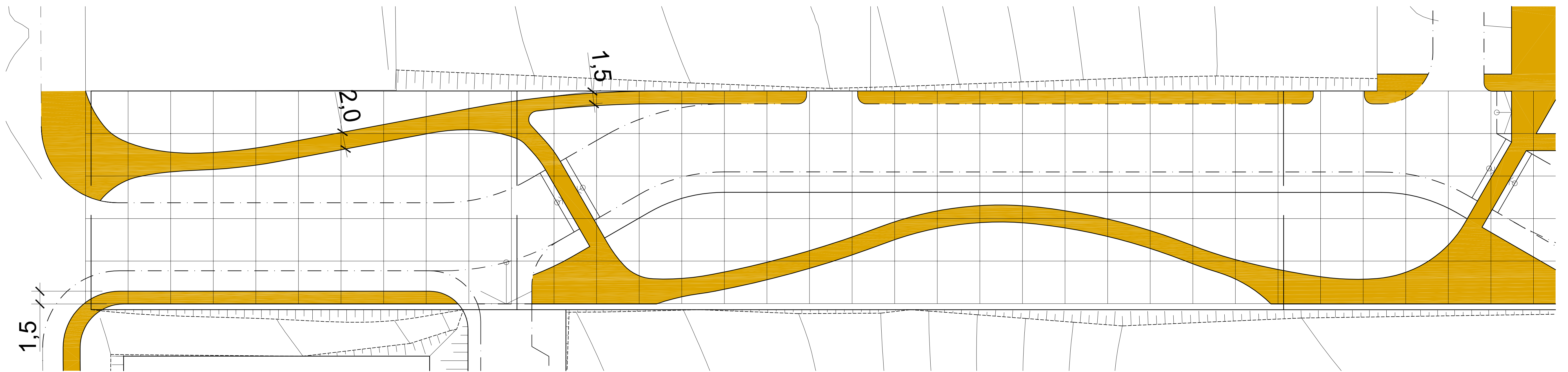
1 Detalhe do Passeio (malha 5x5m) ESCALA 1 : 250
