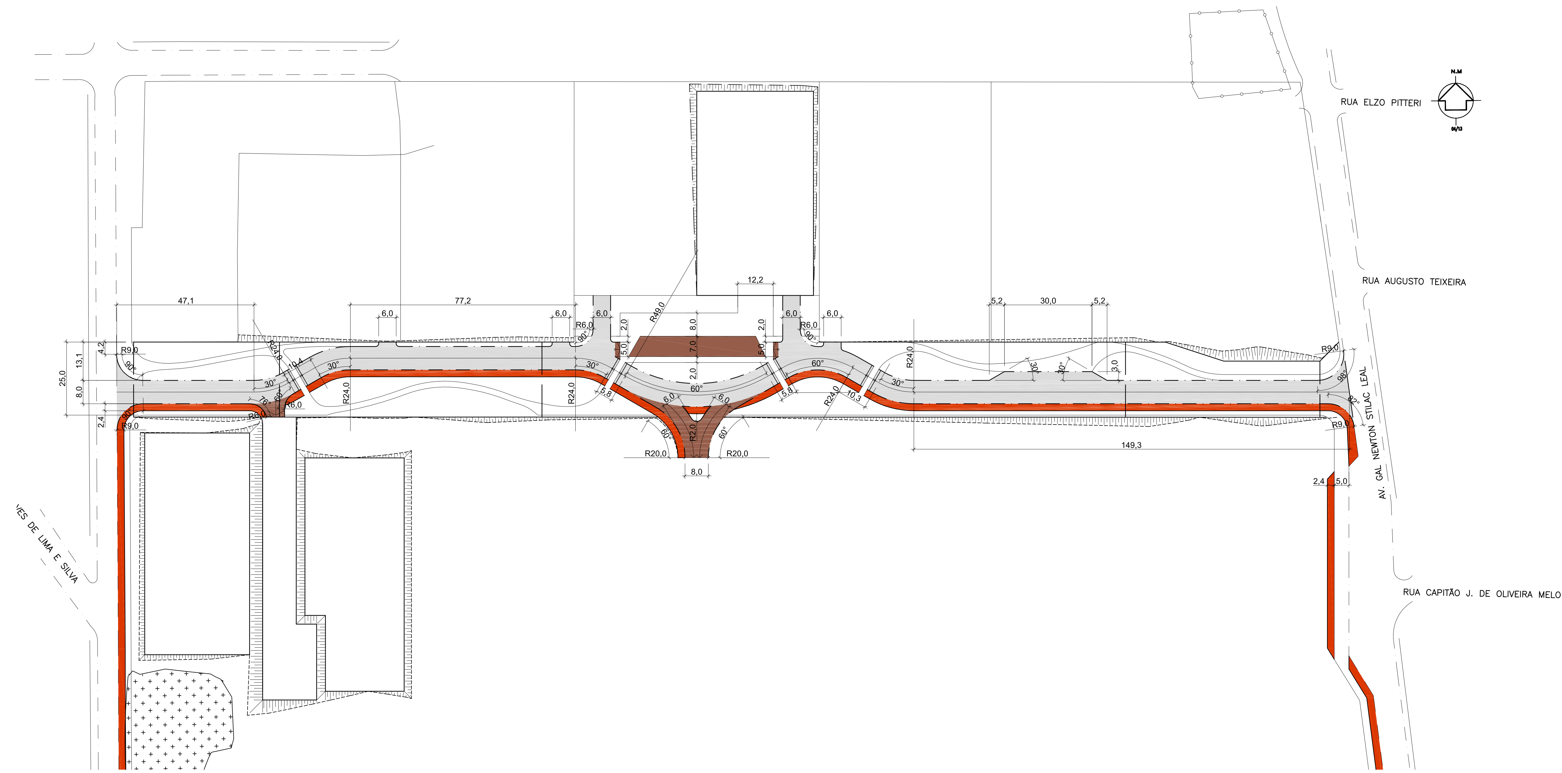
1 Planta de Pavimentação - Leito Carroçável e Ciclovia ESCALA 1 : 750
